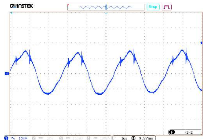
Рис. 40. Пульсации U_{\text{вых.ном}} . Масштаб 10 мВ/дел. Развертка 1 мкс/дел.
