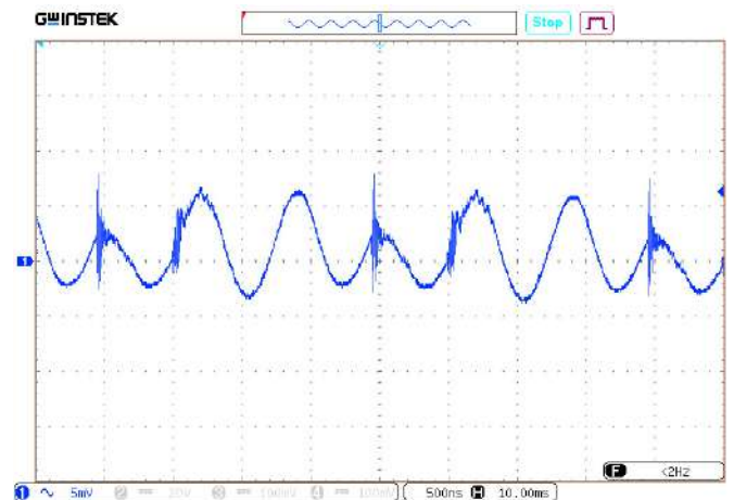
Рис. 44. Пульсации U_{\text{вых.ном}} . Масштаб 5 мВ/дел. Развертка 0,5 мкс/дел.
