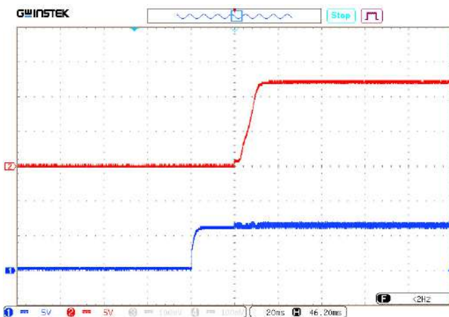
Рис. 37. Установление U_{\text{вых.ном}} с момента подачи сигнала ДУ (соединение выводов «VKЛ» и «-VX»). Луч 1 (синий) – входное напряжение. Масштаб 5 В/дел. Луч 2 (красный) – выходное напряжение. Масштаб 5 В/дел. Развертка 20 мс/дел.
