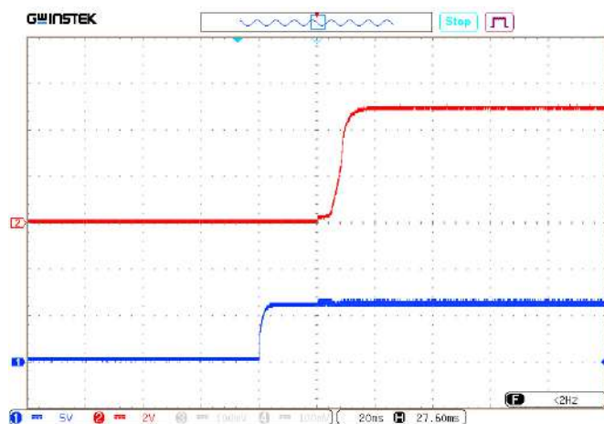
Рис. 29. Установление U_{ВЫХ,НОМ} с момента подачи сигнала ДУ (размыкание выводов «ДУ» и «ВХ»). Луч 1 (синий) – напряжение на выводе «ДУ». Масштаб 5 В/дел. Луч 2 (красный) – выходное напряжение. Масштаб 2 В/дел. Развертка 20 мс/дел.
