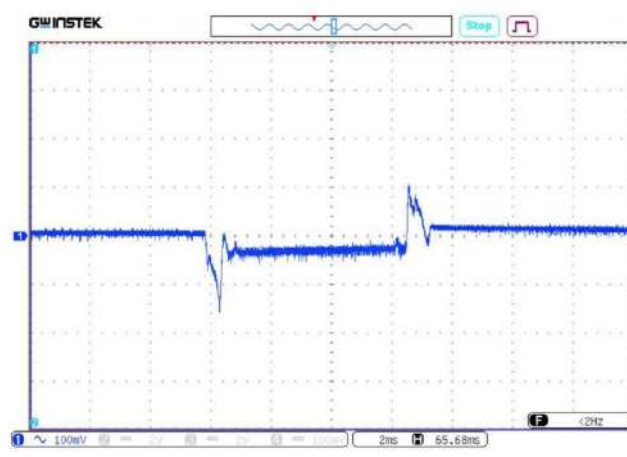
Рис. 30. Осциллограмма переходного отклонения выходного напряжения при скачкообразном изменении выходного тока с 50% до 100% и со 100% до 50%. Масштаб 100 мВ/дел. Развертка 2 мс/дел.
