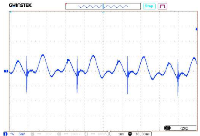
Рис. 32. Осциллограмма пульсаций U_{\text{вых.ном}} . Масштаб 5 мВ/дел. Развертка 1 мкс/дел.
