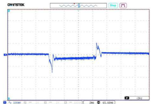
Рис. 42. Осциллограмма переходного отклонения выходного напряжения при скачкообразном изменении выходного тока с 50% до 100% и со 100% до 50%. Масштаб 100 мВ/дел. Развертка 2 мкс/дел.
