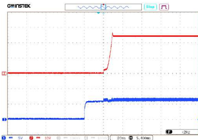
Рис. 33. Установление U_{\text{вых.ном}} с момента подачи сигнала ДУ (соединение выводов «ДУ» и «-ВХ») Луч 1 (синий) – входное напряжение. Масштаб 5 В/дел. Луч 2 (красный) – выходное напряжение. Масштаб 10 В/дел. Развертка 20 мс/дел.
