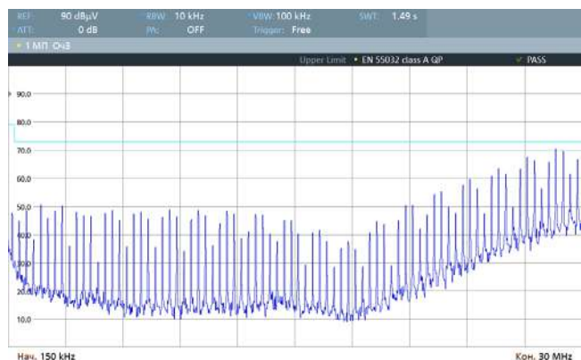
Рис. 45. Спектрограмма работы VDRI30B24 по схеме включения [Рис. 3], измерения произведены в соответствии с EN 55032 Class A (0,15–30 МГц).
