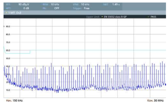
Рис. 42. Спектрограмма работы VDRI20W48 по схеме включения [Рис. 4], измерения произведены в соответствии с EN 55032 Class B (0,15–30 МГц).
