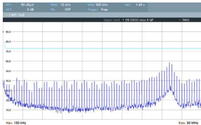
Рис. 43. Спектрограмма работы VDRI30B05 по схеме включения [Рис. 3], измерения произведены в соответствии с EN 55032 Class A (0,15–30 МГц).
