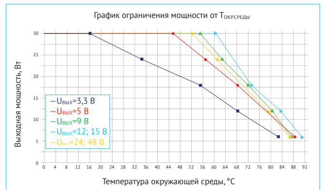
Рис. 26. График ограничения мощности от Tокр.среды без применения внешнего радиатора. Для модулей VDRI30W с входной сетью «W», при U_{ВХ}=48 В .
