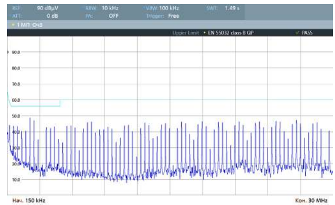
Рис. 40. Спектрограмма работы VDRI20W24 по схеме включения [Рис. 4], измерения произведены в соответствии с EN 55032 Class B (0,15–30 МГц).
