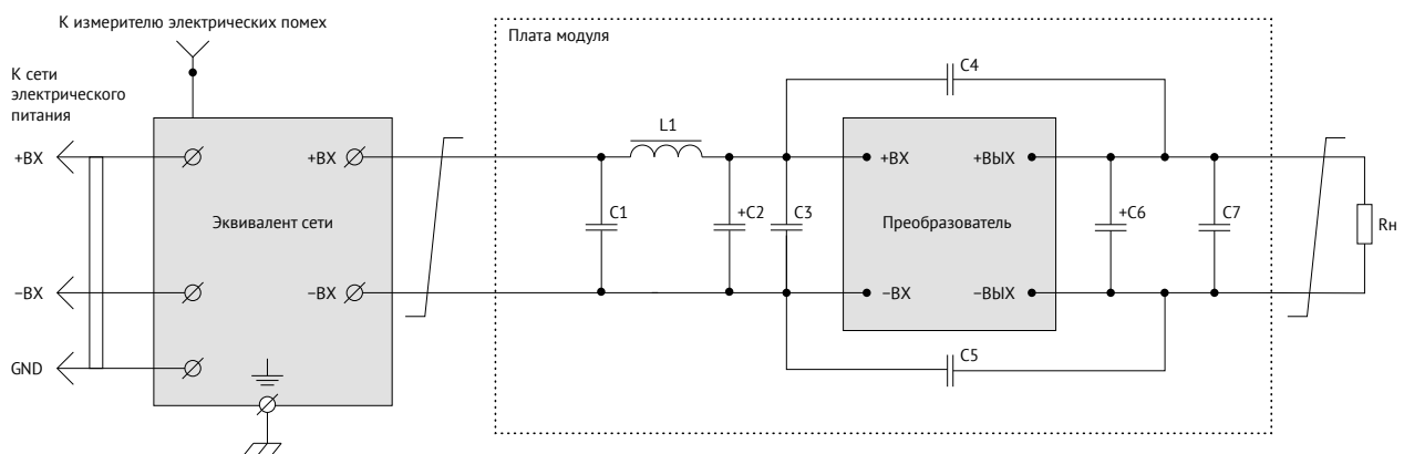
Рис. 3. Схема включения VDRI20, VDRI30 для соответствия стандарту EN 55032 Class A.
