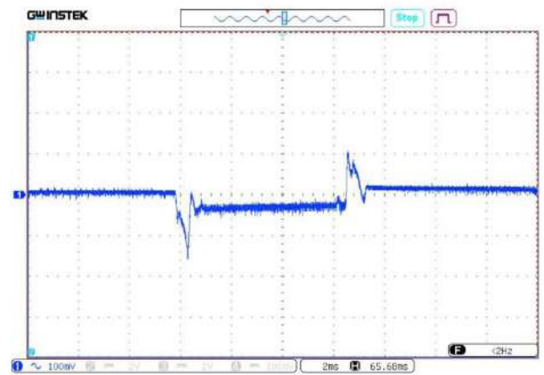
Рис. 32. Осциллограмма переходного отклонения выходного напряжения при скачкообразном изменении выходного тока с 50% до 100% и со 100% до 50%.
