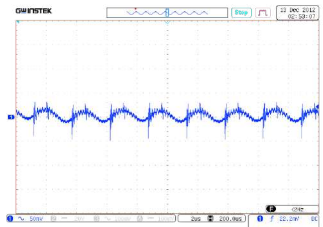
Рис. 35. Пульсации U_{\text{ВЫХ.НОМ}} . Масштаб 10 мВ/дел. Развертка 2 мкс/дел.
