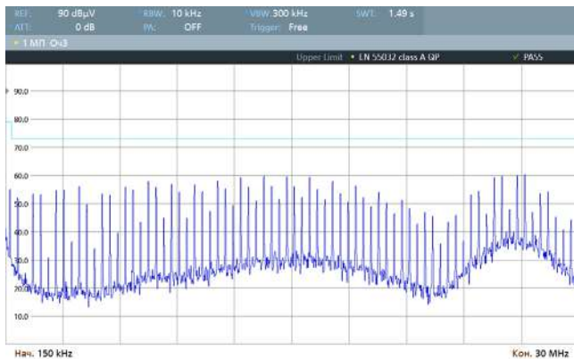
Рис. 44. Спектрограмма работы VDRI60B15 по схеме включения [Рис. 3], измерения произведены в соответствии с EN 55032 Class A (0,15–30 МГц).
