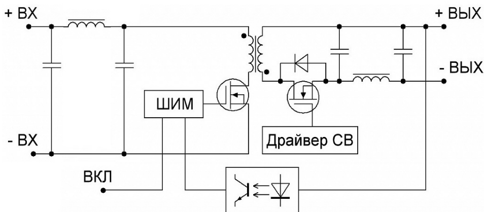
Рис. 1. Функциональная схема VDRI40, VDRI60.
