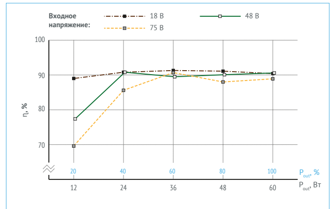
Рис. 20. КПД для VDRI60W15.
