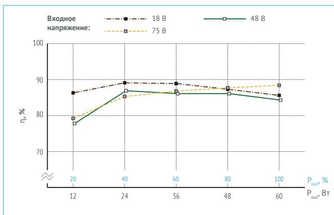
Рис. 17. КПД для VDRI60W05.
