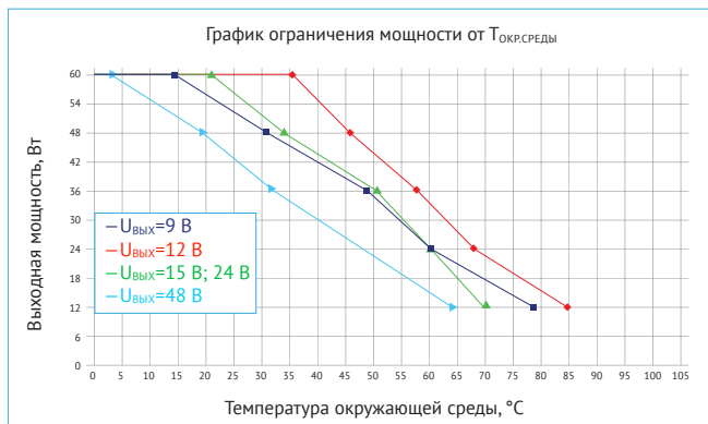
Рис. 22. График ограничения мощности от T_{окр.среды} без применения внешнего радиатора. Для модулей VDRI60B с входной сетью «В», при U_{ВХ}=24 В .
