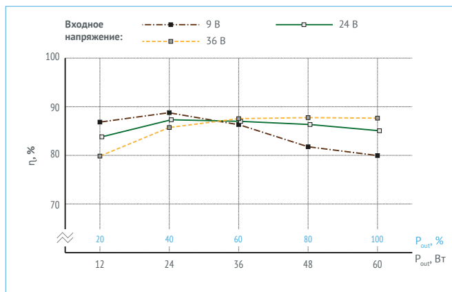
Рис. 11. КПД для VDRI60B05.
