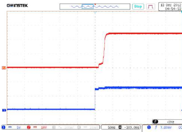
Рис. 36. Установление U_{\text{ВЫХ.НОМ}} с момента подачи сигнала ДУ (соединение выводов «ВКЛ» и «ВХ».) Луч 1 (синий) – входное напряжение. Масштаб 5 В/дел. Луч 2 (красный) – выходное напряжение. Масштаб 10 В/дел. Развертка 50 мс/дел.
