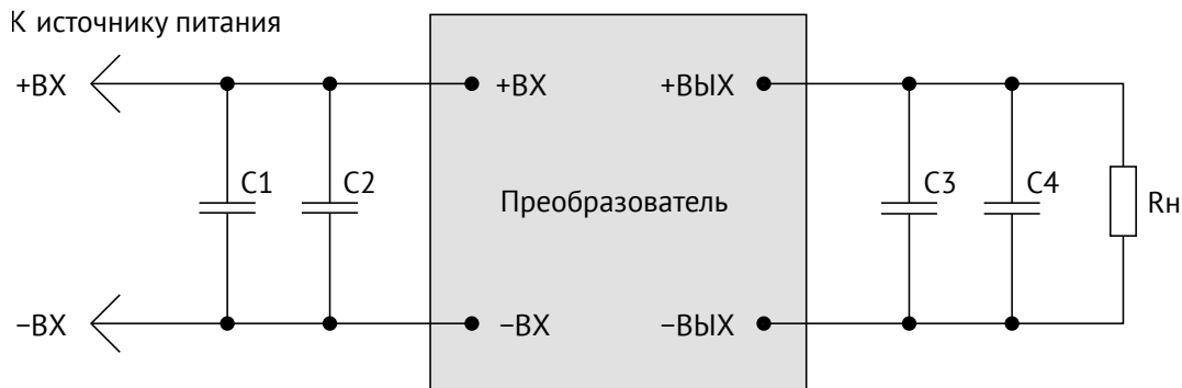
Рис. 2. Типовая схема включения VDRI40, VDRI60.
