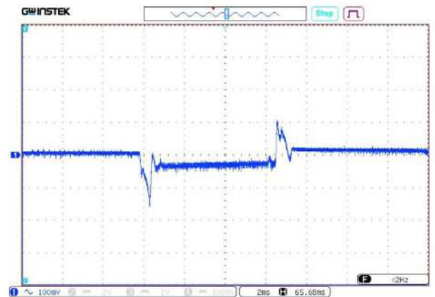
Рис. 37. Осциллограмма переходного отклонения выходного напряжения при скачкообразном изменении выходного тока с 50% до 100% и со 100% до 50%. Масштаб 100 мВ/дел. Развертка 2 мкс/дел.
