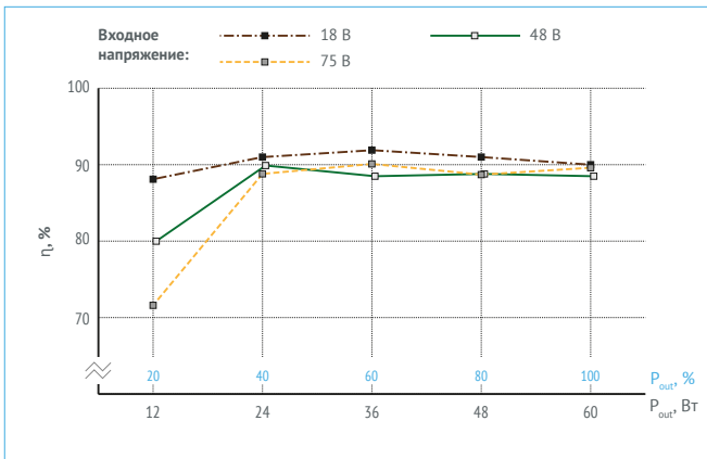
Рис. 19. КПД для VDRI60W12.
