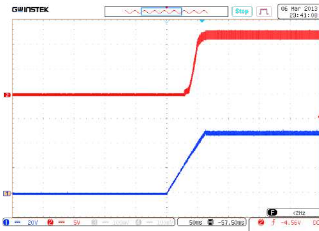
Рис. 30. Установление U_{\text{вых.ном}} с момента подачи U_{\text{вх.ном}} . Луч 1 (синий) – входное напряжение. Масштаб 20 В/дел. Луч 2 (красный) – выходное напряжение. Масштаб 5 В/дел. Развертка 50 мс/дел.
