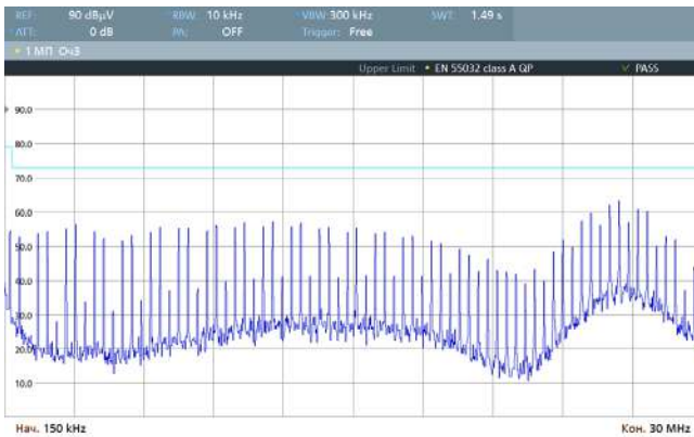
Рис. 40. Спектрограмма работы VDRI40B15 по схеме включения [Рис. 3], измерения произведены в соответствии с EN 55032 Class A (0,15–30 МГц).
