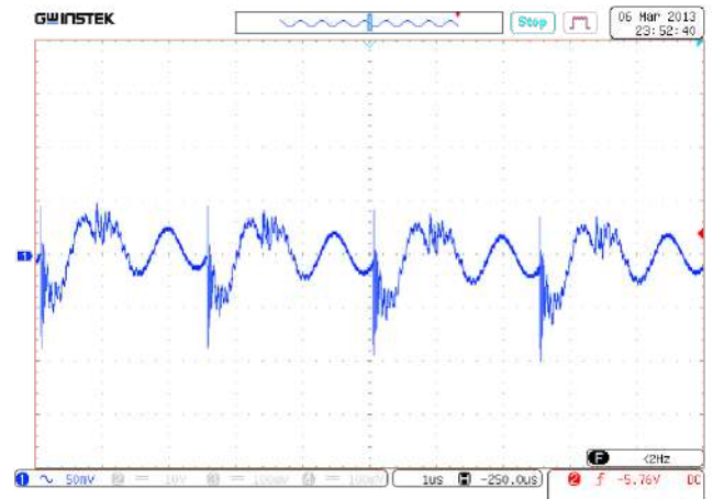
Рис. 31. Пульсации U_{\text{вых.ном}} . Масштаб 50 мВ/дел. Развертка 1 мкс/дел.
