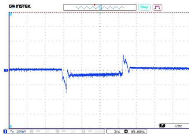
Рис. 25. Осциллограмма переходного отклонения выходного напряжения при скачкообразном изменении выходного тока с 50% до 100% и со 100% до 50%. Масштаб 100 мВ/дел. Развертка 2 мс/дел.
