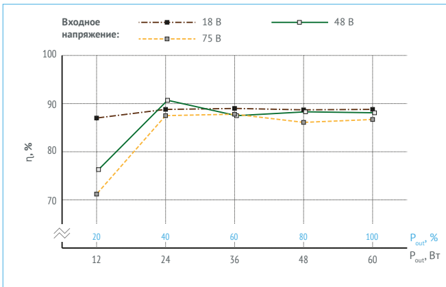
Рис. 21. КПД для VDRI60W24.
