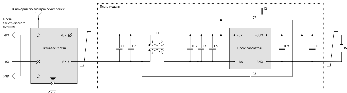
Рис. 4. Схема включения VDRI40, VDRI60 для соответствия стандарту EN 55032 Class B.
