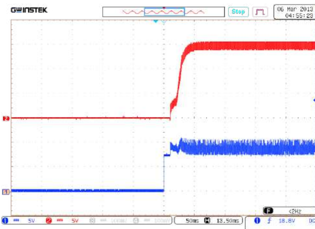
Рис. 24. Установление U_{ВЫХ.НОМ} с момента подачи сигнала ДУ (размыкание выводов «ДУ» и «ВХ»). Луч 1 (синий) — напряжение на выводе «ДУ». Масштаб 5 В/дел. Луч 2 (красный) — выходное напряжение. Масштаб 5 В/дел. Развертка 50 мс/дел.
