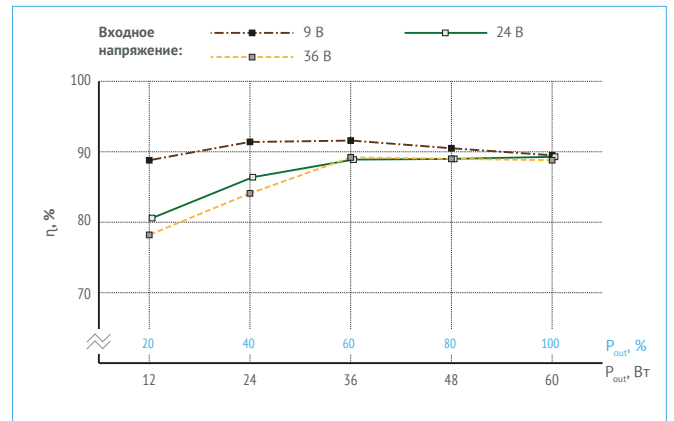
Рис. 14. КПД для VDRI60B15.
