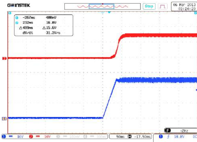
Рис. 26. Установление U_{\text{ВЫХ.НОМ}} с момента подачи U_{\text{ВХ.НОМ}} . Луч 1 (синий) – входное напряжение. Масштаб 10 В/дел. Луч 2 (красный) – выходное напряжение. Масштаб 10 В/дел. Развертка 50 мс/дел.
