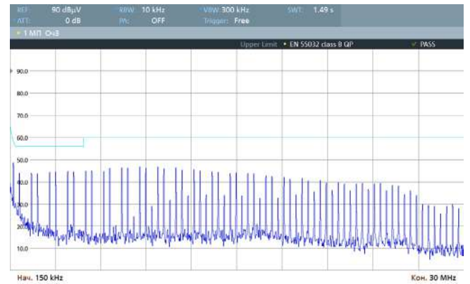
Рис. 43. Спектрограмма работы VDRI40W15 по схеме включения [Рис. 4], измерения произведены в соответствии с EN 55032 Class B (0,15–30 МГц).
