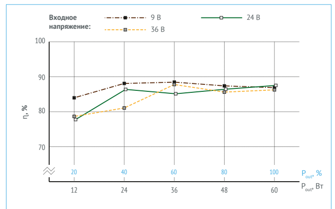
Рис. 16. КПД для VDRI60B48.
