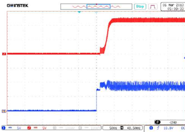
Рис. 28. Установление U_{\text{ВЫХ.НОМ}} с момента подачи сигнала ДУ (соединение выводов «ДУ» и «-ВХ».) Луч 1 (синий) – входное напряжение. Масштаб 5 В/дел. Луч 2 (красный) – выходное напряжение. Масштаб 5 В/дел. Развертка 50 мс/дел.
