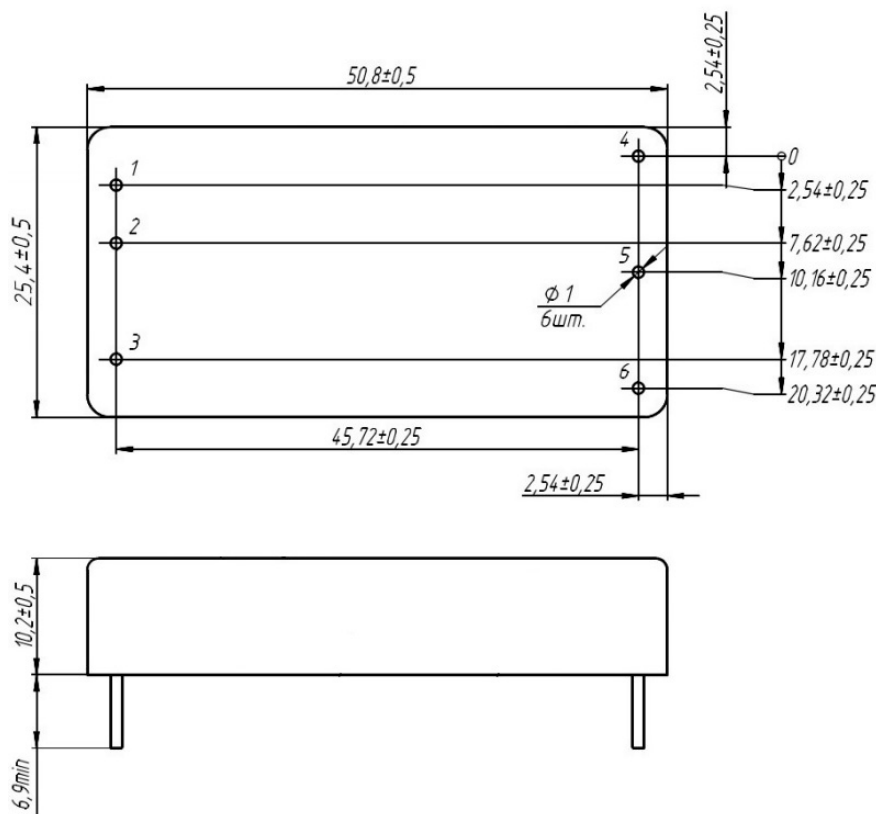
Рис. 48. Исполнение VDRI40, VDRI60.
