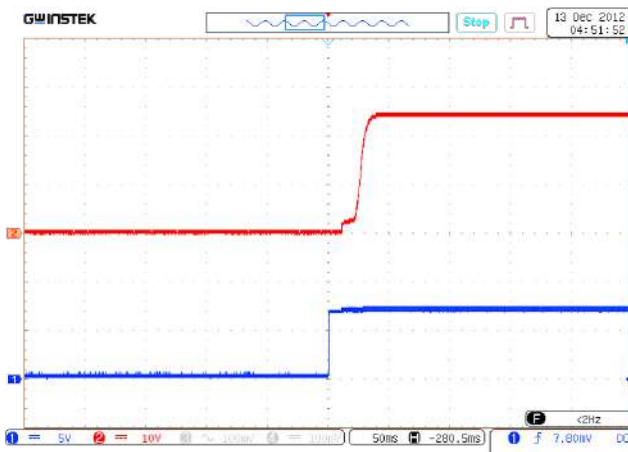
Рис. 32. Установление U_{\text{вых.ном}} с момента подачи сигнала ДУ (соединение выводов «ВКЛ» и «-ВХ».) Луч 1 (синий) – входное напряжение. Масштаб 5 В/дел. Луч 2 (красный) – выходное напряжение. Масштаб 10 В/дел. Развертка 50 мс/дел.
