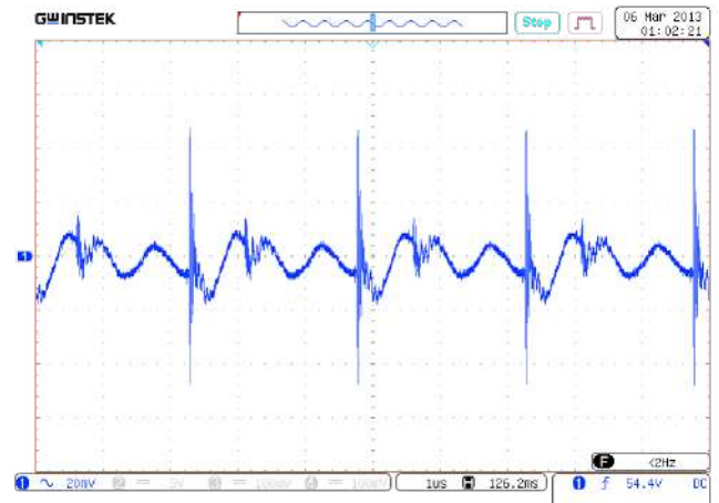
Рис. 27. Осциллограмма пульсаций U_{\text{ВЫХ.НОМ}} . Масштаб 20 мВ/дел. Развертка 1 мкс/дел.
