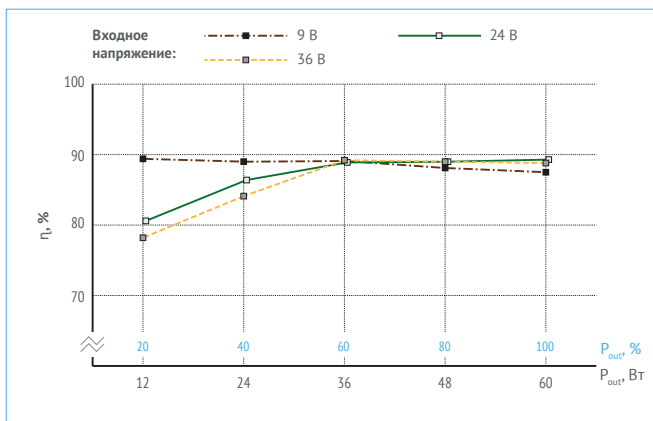
Рис. 15. КПД для VDRI60B24.
