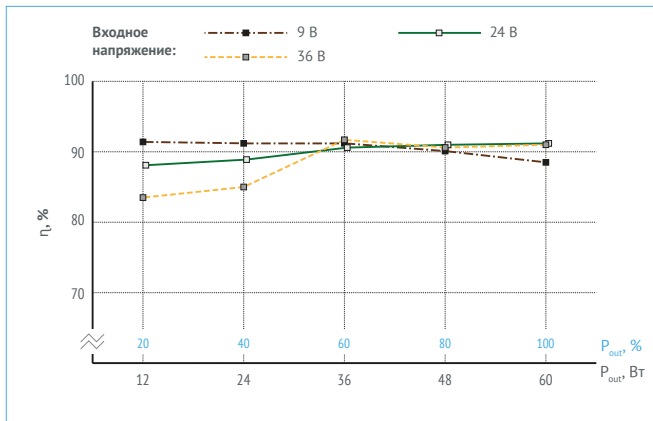
Рис. 13. КПД для VDRI60B12.
