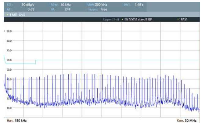
Рис. 41. Спектрограмма работы VDRI40B15 по схеме включения [Рис. 4], измерения произведены в соответствии с EN 55032 Class B (0,15–30 МГц).
