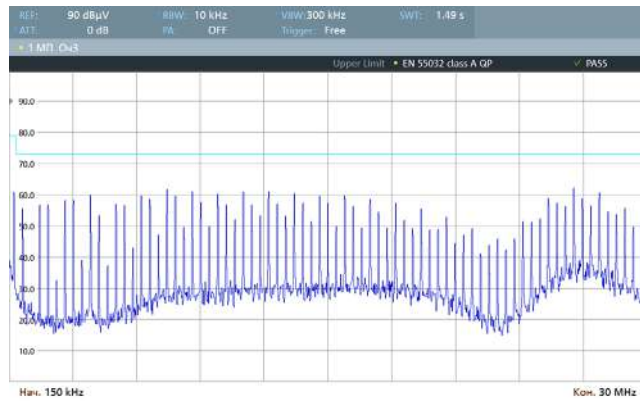
Рис. 46. Спектрограмма работы VDRI60W15 по схеме включения [Рис. 3], измерения произведены в соответствии с EN 55032 Class A (0,15–30 МГц).
