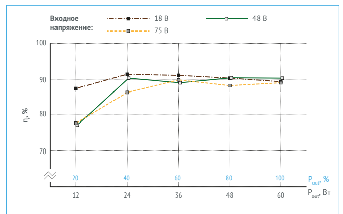
Рис. 18. КПД для VDRI15W09.
