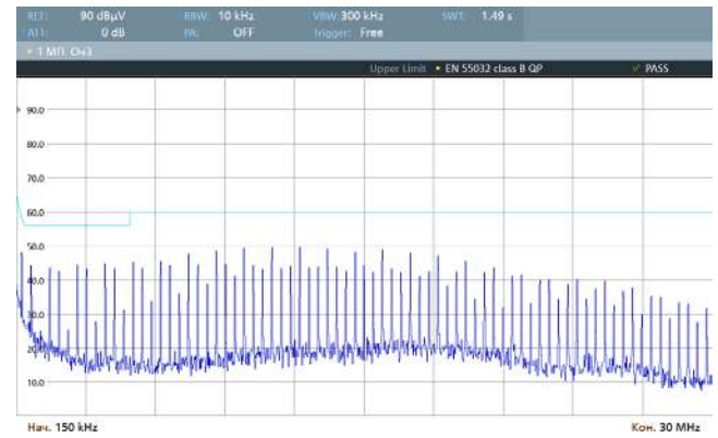
Рис. 47. Спектрограмма работы VDRI60W15 по схеме включения [Рис. 4], измерения произведены в соответствии с EN 55032 Class B (0,15–30 МГц).
