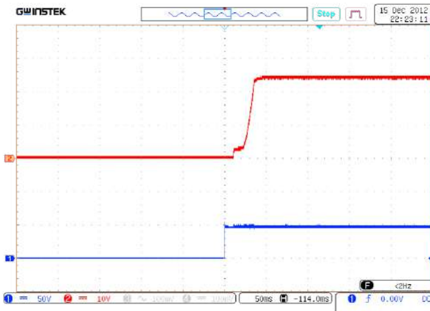
Рис. 38. Установление U_{\text{вых.ном}} с момента подачи U_{\text{вх.ном}} . Луч 1 (синий) – входное напряжение. Масштаб 50 В/дел. Луч 2 (красный) – выходное напряжение. Масштаб 10 В/дел. Развертка 50 мс/дел.
