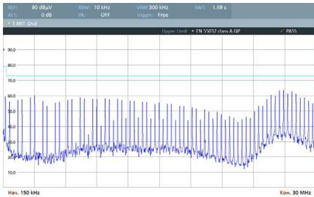
Рис. 42. Спектрограмма работы VDRI40W15 по схеме включения [Рис. 3], измерения произведены в соответствии с EN 55032 Class A (0,15–30 МГц).
