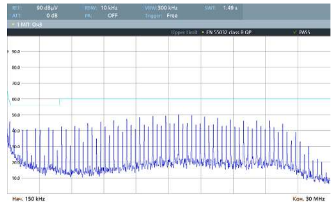
Рис. 45. Спектрограмма работы VDRI60B15 по схеме включения [Рис. 4], измерения произведены в соответствии с EN 55032 Class B (0,15–30 МГц).
