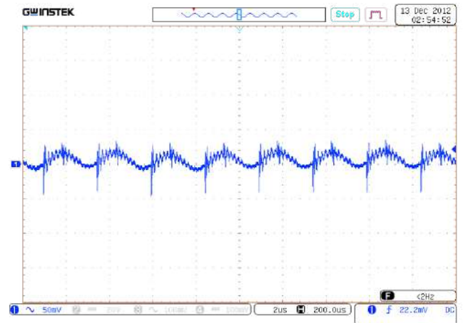
Рис. 39. Пульсации U_{\text{вых.ном}} . Масштаб 50 мВ/дел. Развертка 2 мкс/дел.
