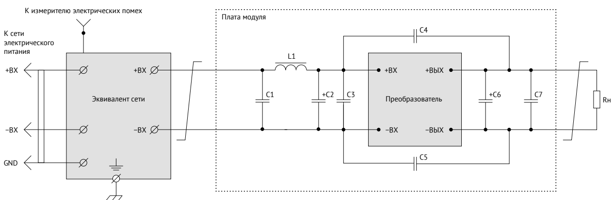
Рис. 3. Схема включения VDRI40, VDRI60 для соответствия стандарту EN 55032 Class A.
