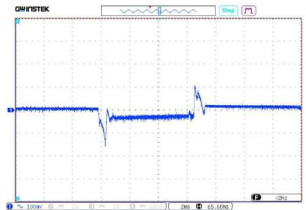
Рис. 33. Осциллограмма переходного отклонения выходного напряжения при скачкообразном изменении выходного тока с 50% до 100% и со 100% до 50%. Масштаб 100 мВ/дел. Развертка 2 мкс/дел.
