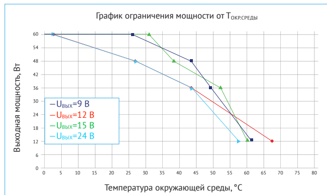
Рис. 23. График ограничения мощности от T_{окр.среды} без применения внешнего радиатора. Для модулей VDRI60W с входной сетью «W», при U_{ВХ}=48 В .
