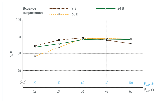
Рис. 12. КПД для VDRI60B09.
