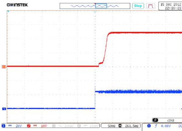
Рис. 34. Установление U_{\text{ВЫХ.НОМ}} с момента подачи U_{\text{ВХ.НОМ}} . Луч 1 (синий) – входное напряжение. Масштаб 20 В/дел. Луч 2 (красный) – выходное напряжение. Масштаб 10 В/дел. Развертка 50 мс/дел.
